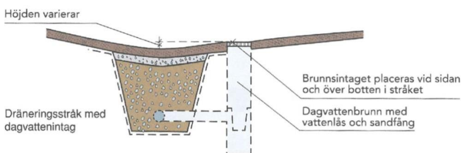
Figur 1. Makadamfyllt infiltrationsstråk med dagvattenintag. Bildkälla: Svenskt Vatten, 2011.
