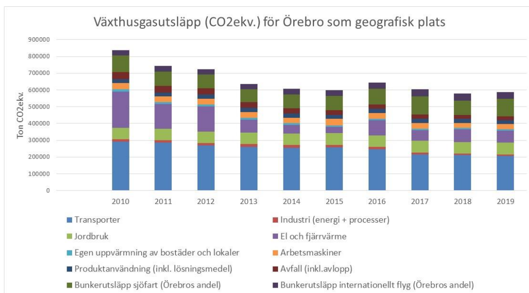
Figur 7, Växthusgasutsläpp hämtade från nationella emissionsdatabasen, regional utveckling och samverkan i miljömålsystemet (RUS), samt Örebro kommuns andel av utsläpp från utrikes flyg och sjöfart (bunkerutsläpp, SCB).
