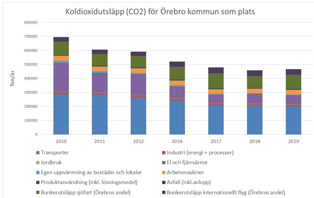
Figur 6, Koldioxidutsläpp från nationella emissionsdatabasen, regional utveckling och samverkan i miljömålssystemet (RUS), samt Örebro kommuns andel av utsläpp från utrikes flyg och sjöfart (bunkerutsläpp, SCB).
