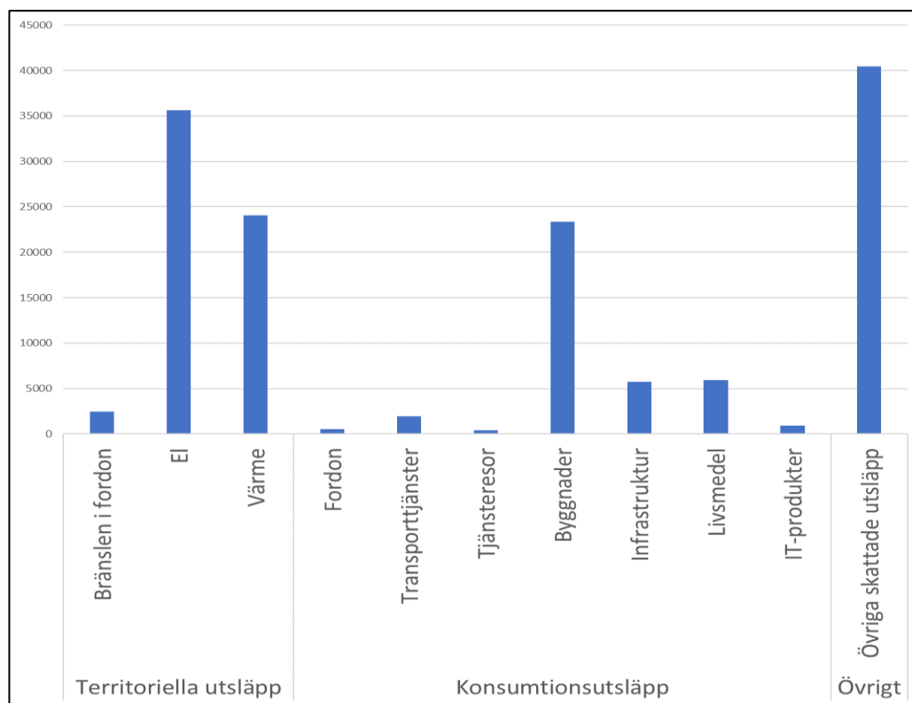
Figur 8, Utsläpp kategoriserade som territoriella och konsumtionsbaserade, för Örebro kommunkoncern. Kategorin "Byggnader" avser byggnationsprocessen.
